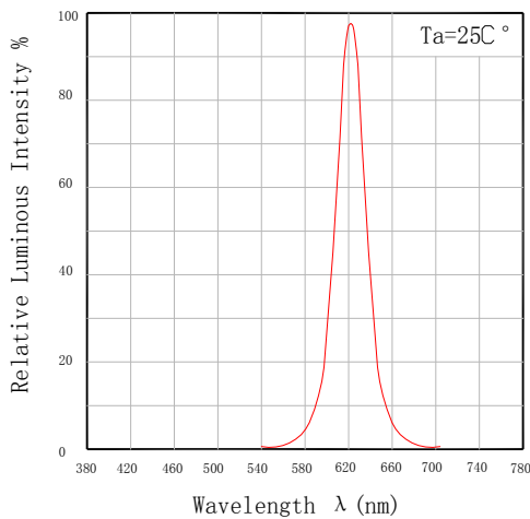
光谱特性图
