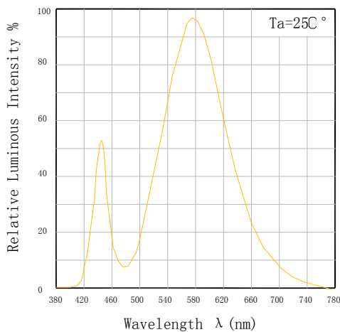
光谱特性图
