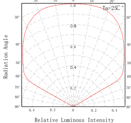
发光角度图
