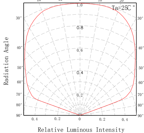
发光角度图
