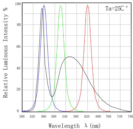
光谱特性图
