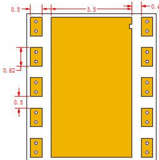
背面图
