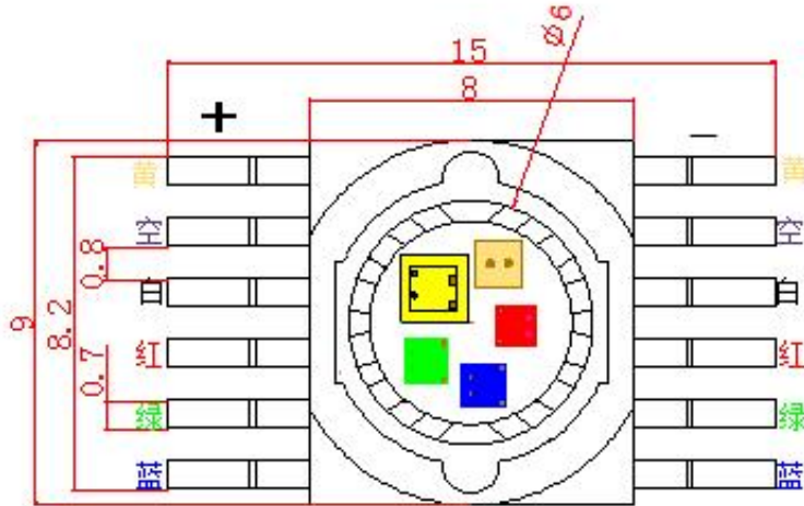
俯视图
