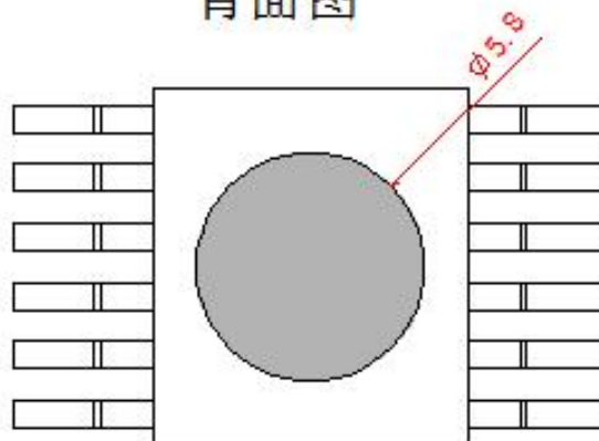
背面图
