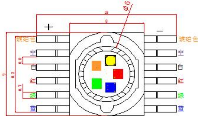
俯视图
