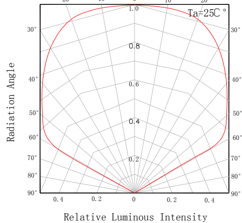
发光角度图
