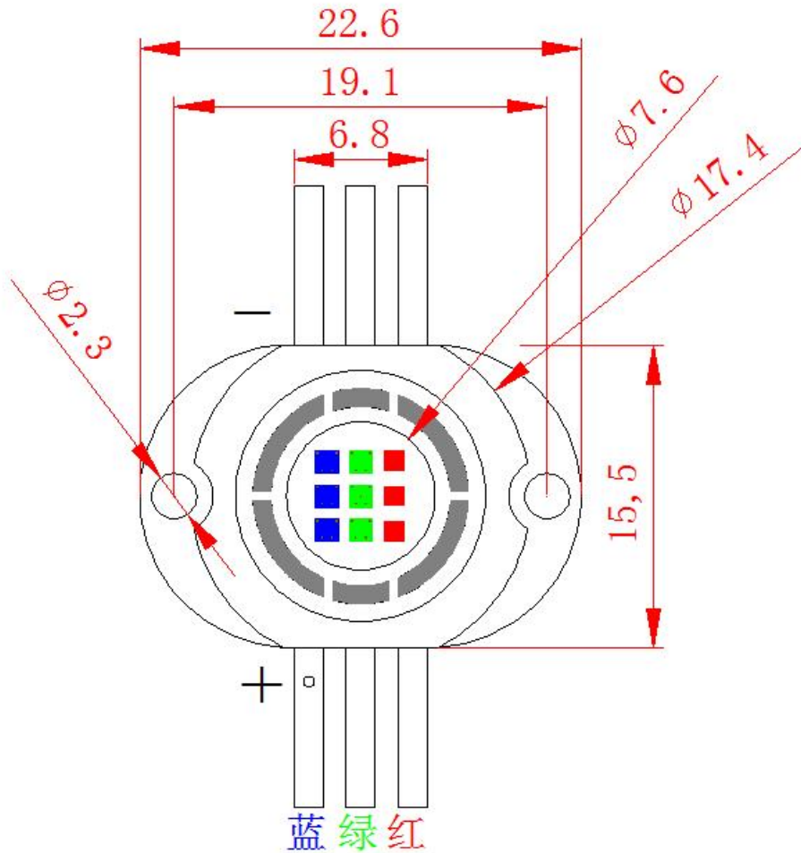
俯视图
