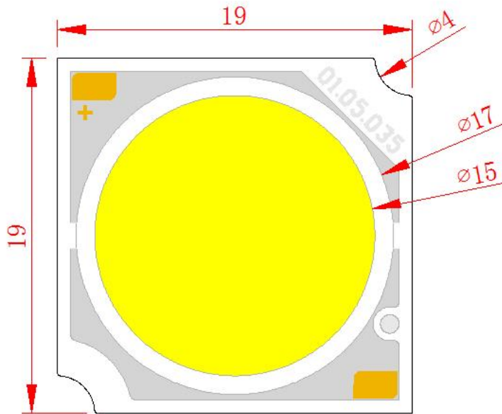
俯视图
