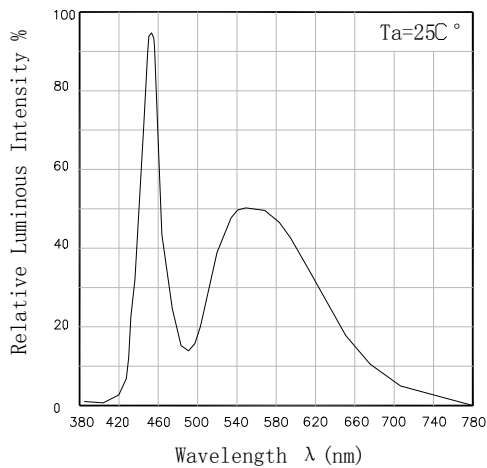
光谱特性图
