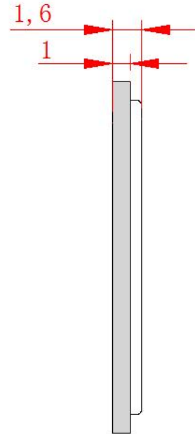
侧视图
