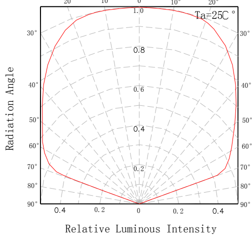
发光角度图
