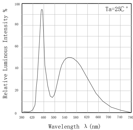
光谱特性图
